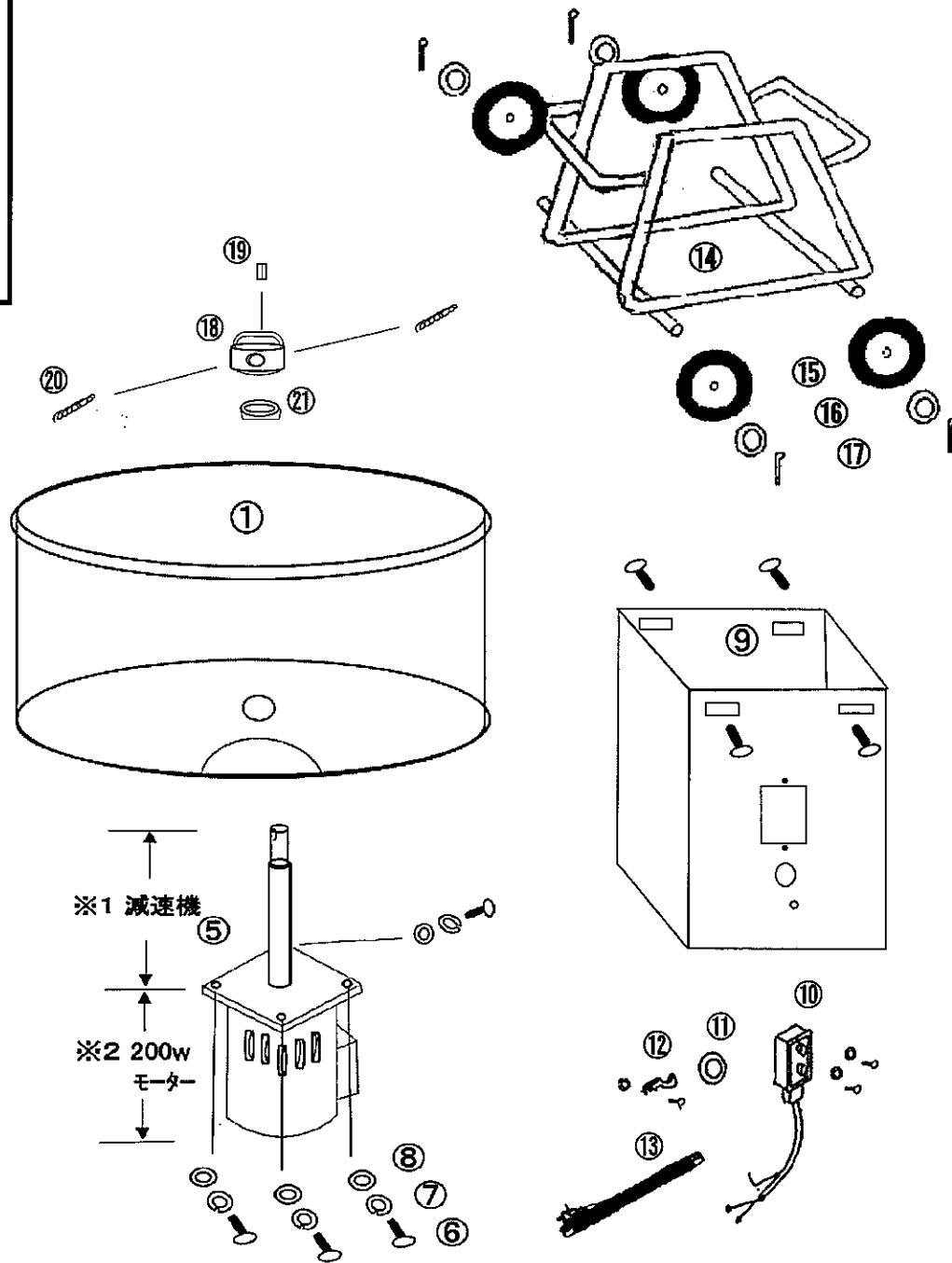
EMG-S1.5B 分解図
