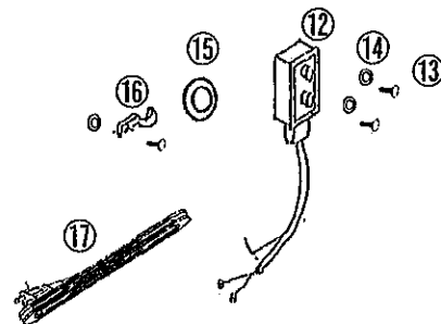
EMG-2.5H 分解図
