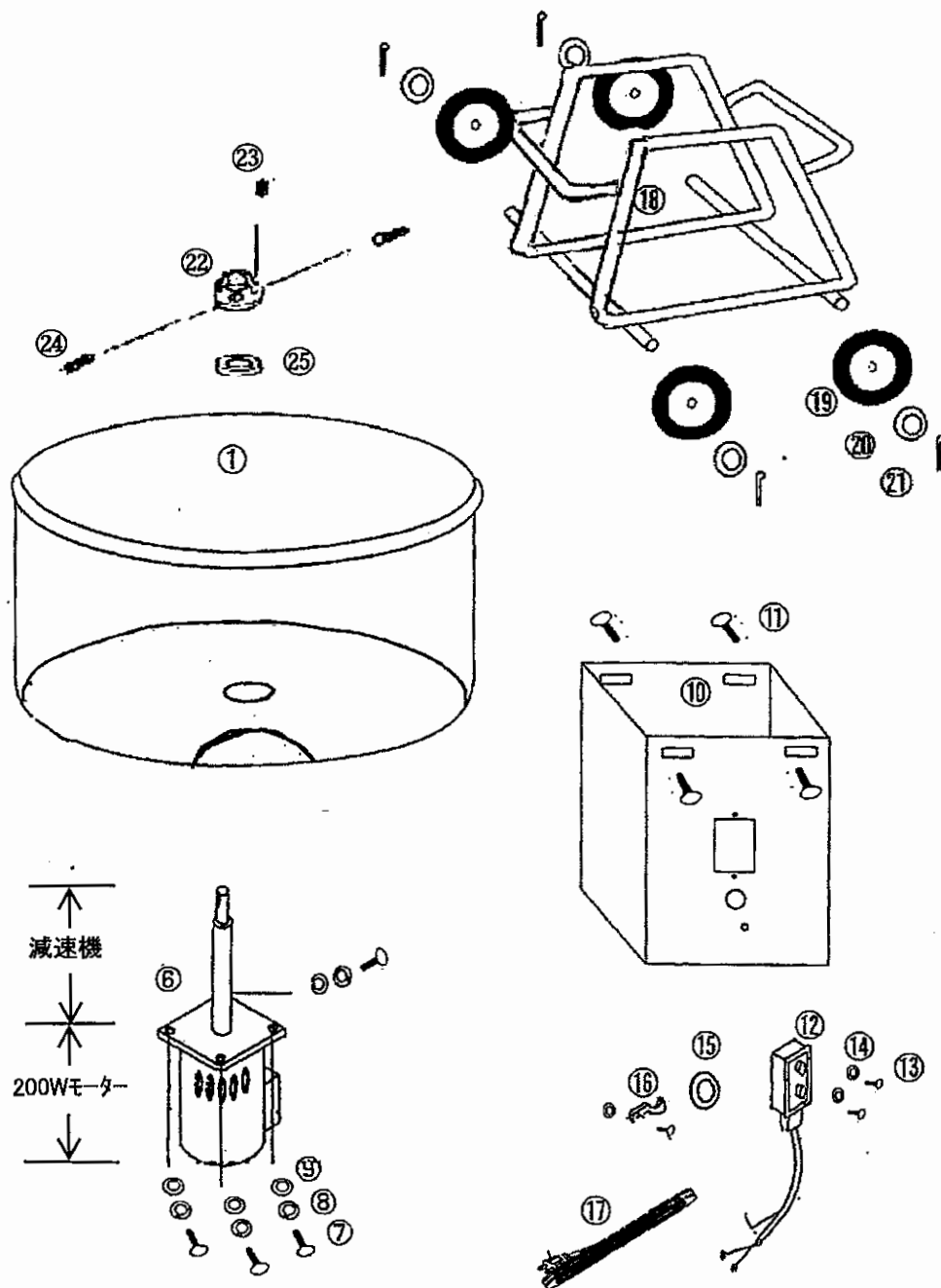
EMG-S1.5B 分解図
