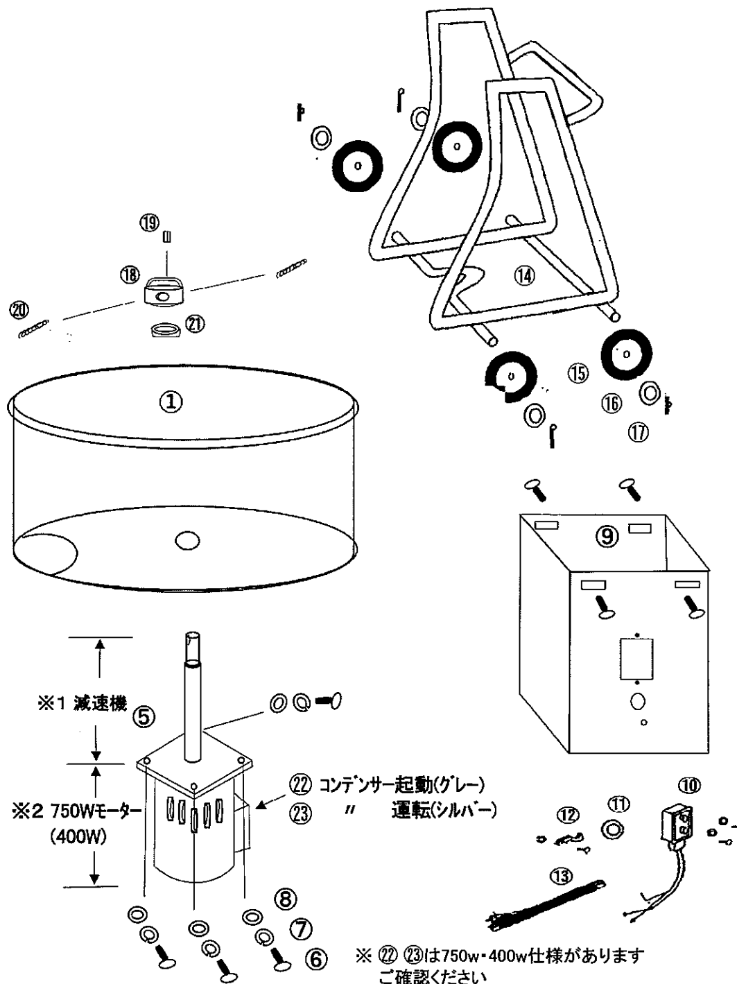
EMG-2.5H 分解図
