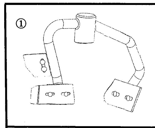
EMG-2.5型羽根軸（完成羽根軸） 分解図 (H, HT含む)
