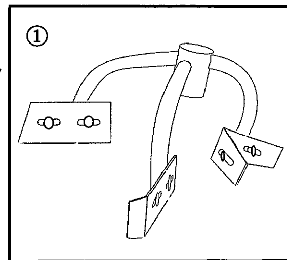
EMG-T25羽根軸 (完成羽根軸) 分解図 (L. H. HSS含む)
